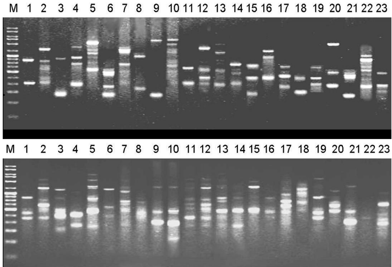
Figure 1. ISSR banding pattern of 23 species/ variety of Ficus using synthesis primer (GA)_8A [A] and (TG)_8A [B]. M –low range DNA marker. F1: Ficus religiosa , F2: Ficus microcarpa “Microcarpa”, F3: Ficus elastica “Rubra”, F4: Ficus repens , F5: F. krisnae , F6: F. elmira , F7: F. petiolaris , F8: F. nervosa , F9: F. microcarpa “Varigatae”, F10: F. benjamina “Varigatae”, F11: F. elastica “Robusta”, F12: F. elastica “varigatae”, F13: F. mollis , F14: F. callosa , F15: F. rumphii “Varigatae”, F16: F. benjimina “Nuda”, F17: F. glomerata , F18: F. virens “Glabella”, F19: F. arnottina , F20: F. bhengalensis , F21: F. amplissima , F22: F. virens “Virens”, F23: F. macrophylla .
